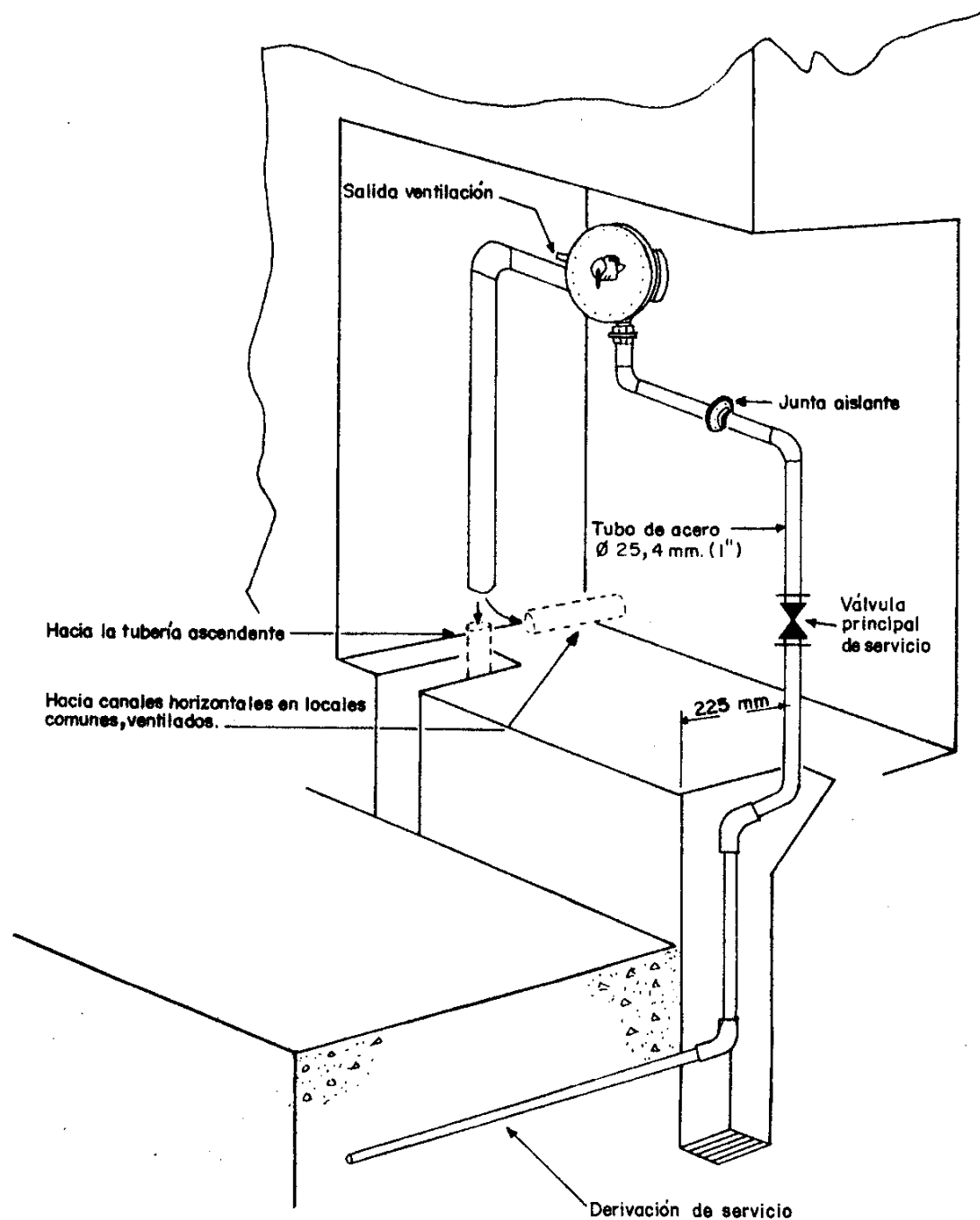
FIGURA Nº 8 CASETA DE REGULACION EMPOTRADA
